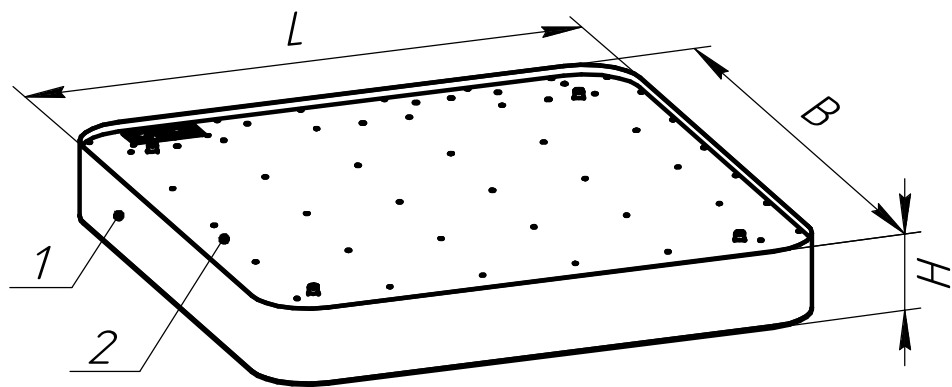
Рисунок 1 - Светильник серии ДСО33 Horizon Four 1 - корпус со встроенным рассеивателем, 2 - панель со встроенным светодиодным модулем и источником питания
