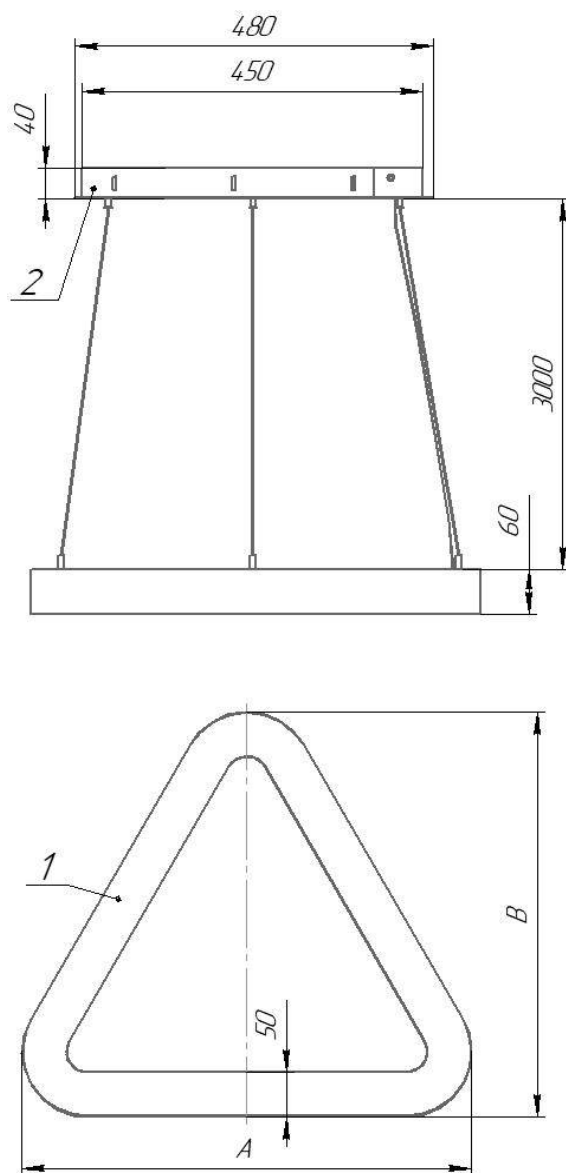
Рисунок 1 - Общий вид светильников серии ДСО33 Horizon Toro
