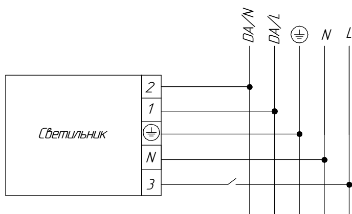
Рисунок 4 - Схема подключения светильников
