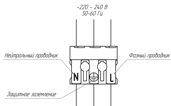
Рис. 3 Схема подключения.
