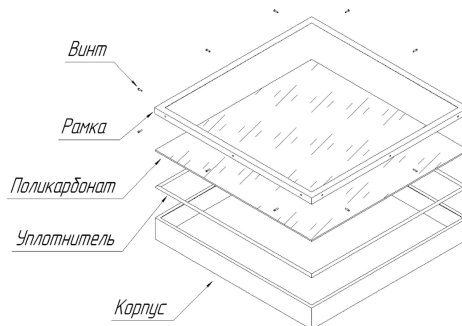
Рис. 2 Взрыв-схема.
