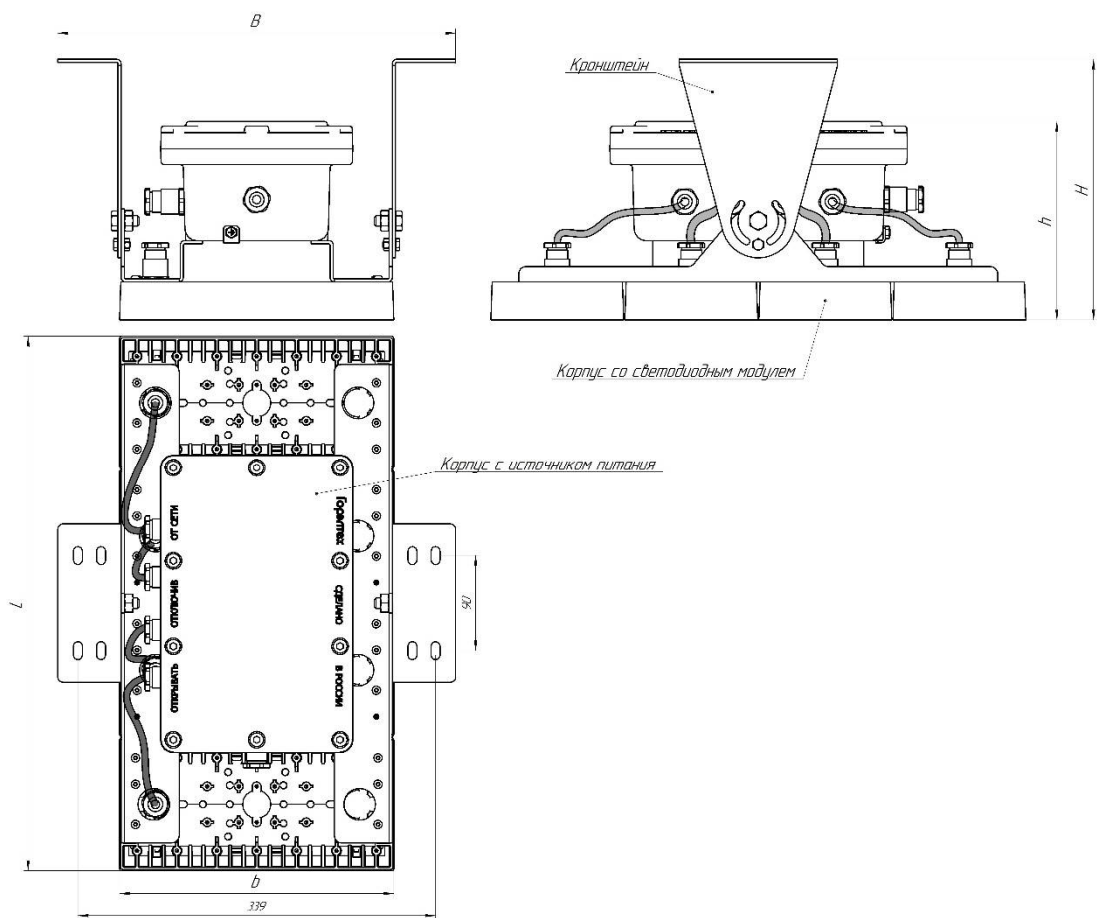
Рисунок 4 - Габаритные размеры светильника ДСП36-210.
