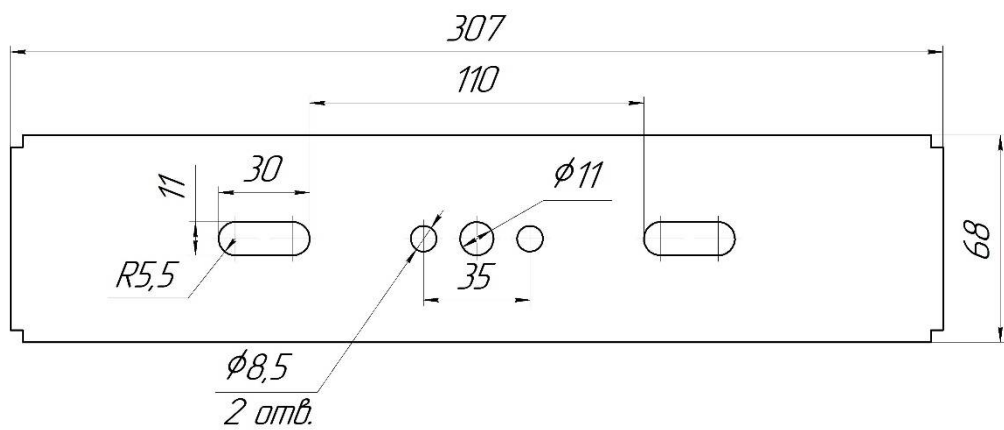
Рисунок 11 - Лира светильника (35-55 Вт).
