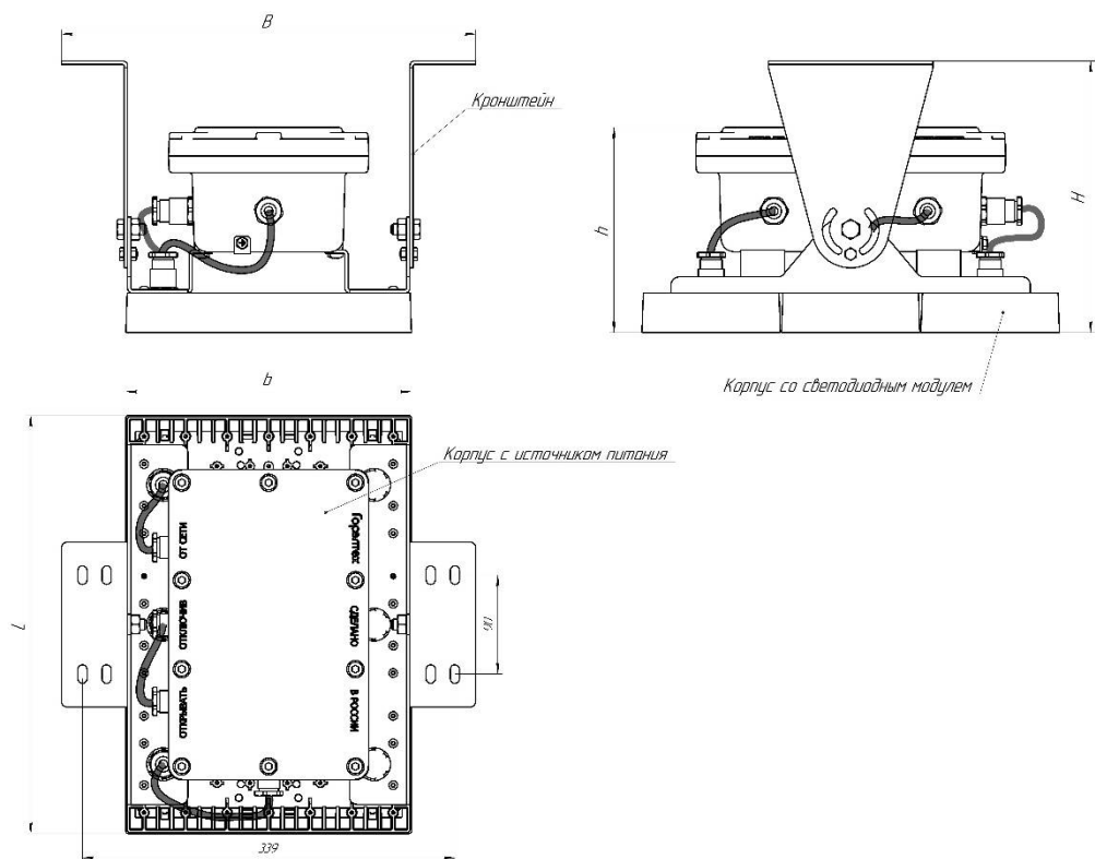
Рисунок 3 - Габаритные размеры светильника ДСП36-160 (ЕМ3).
