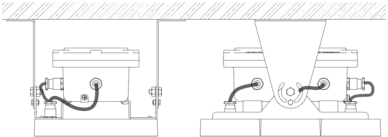
Рисунок 9 - Схема установки светильника (35-55 Вт) на потолок (стену).
