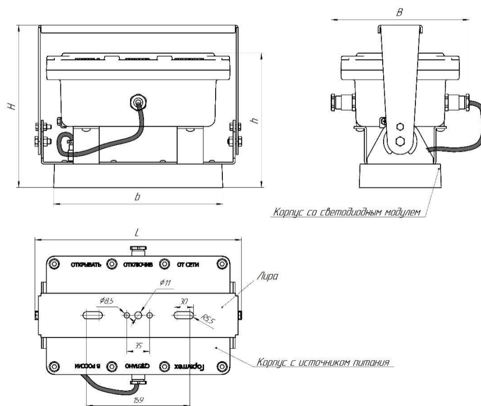
Рисунок 1 - Габаритные размеры светильника ДСП36-35, 55 (ЕМЗ).
