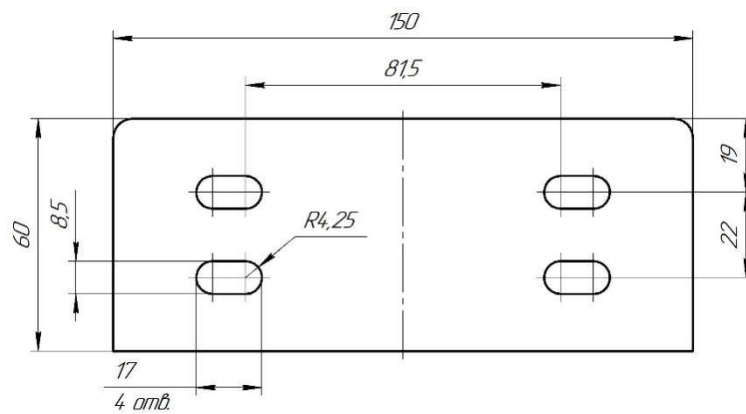
Рисунок 12 - Кронштейн светильника (110-270 Вт).
