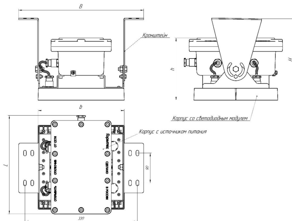
Рисунок 2 - Габаритные размеры светильника ДСП36-110 (ЕМЗ).
