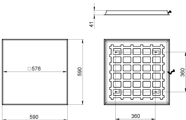
Рис.1 Габаритный чертеж.
