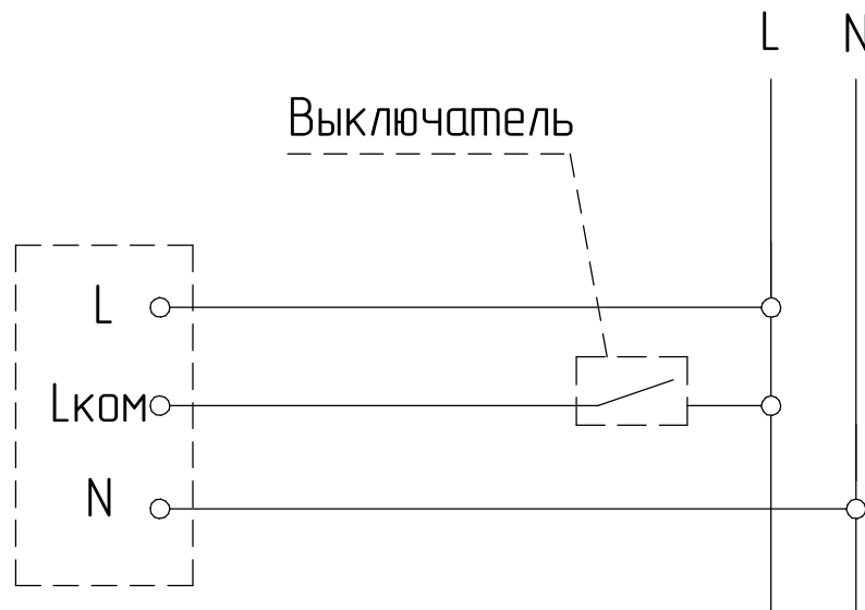
Рисунок 4 - Схема подключения светильника с БАП и II классом защиты к сети.
