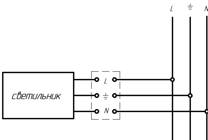
Рисунок 3 - Схема подключения светильников к сети
