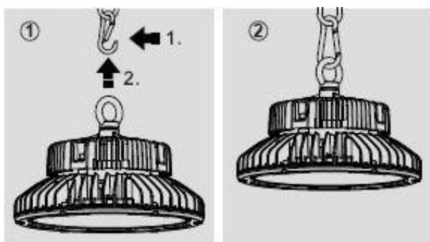
Рисунок 2 - Монтаж светильников с рым болтом
