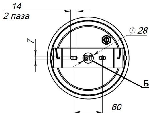
Установочные размеры
