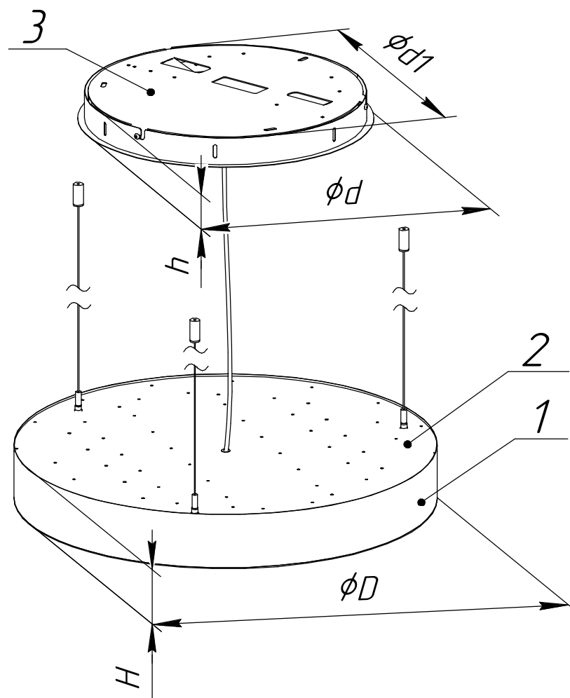
Рисунок 1 - Светильник серии ДСО33 Horizon Sun
