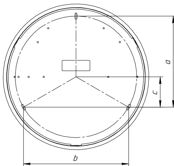
Рисунок 3.2 - Схема нанесения разметки для установки отсека светильника Horizon Sun
