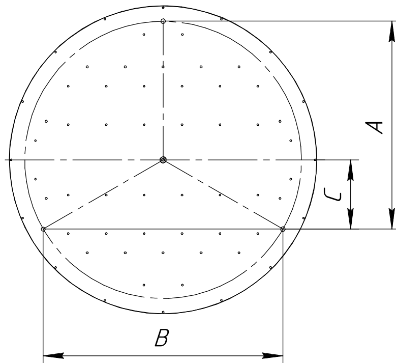
Рисунок 3.1 - Схема нанесения разметки для установки подвесов светильника Horizon Sun.
