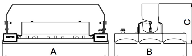
Габариты светильника
