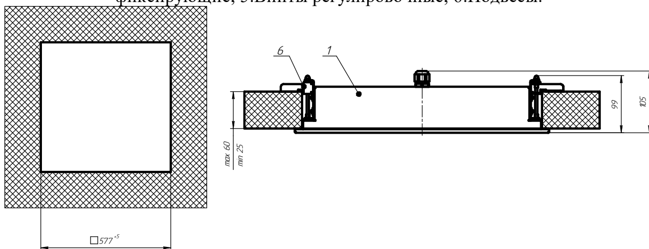
Рис.2.1 Установка светильника.
