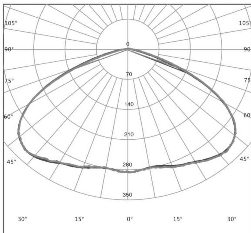
Рисунок 5 - КСС световизлучающего модуля ДБАП02.
