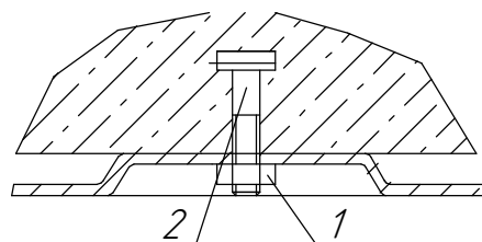
Рисунок 6. Крепление светильника на монтажную поверхность. 1.Гайка.2.Болт.
