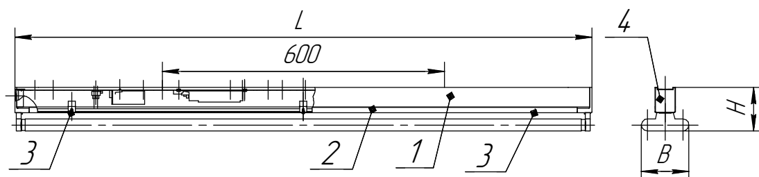
Рисунок 4. 1 - Корпус в сборе, 2 - Крышка, 3 - Винт, 4 - Крышка.
