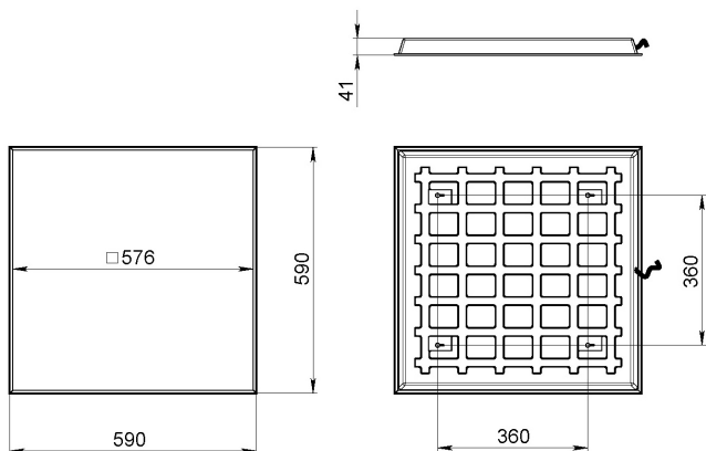
Рис.1 Габаритный чертёж.
