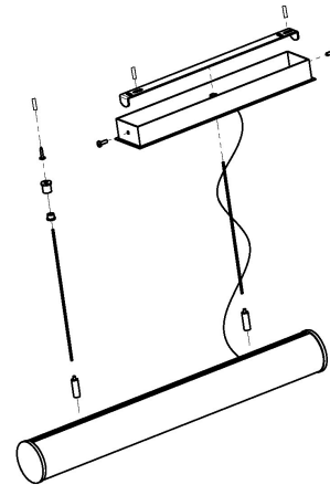
Рис. 2 Монтажный чертеж.
