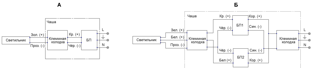
Рис. 3. Схема монтажных соединений. (Рисунок 3А для Д2=310 мм; Рисунок 3Б для Д2=600 мм.)
