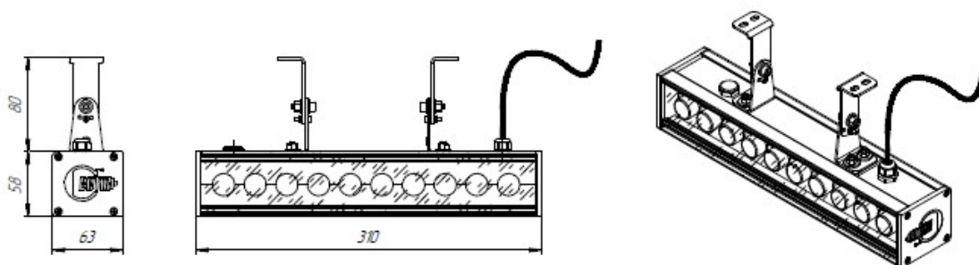
Рис.1 Габаритные размеры.
