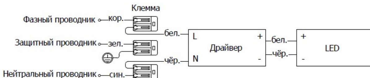
Рис.2 Принципиальная схема подключения.
