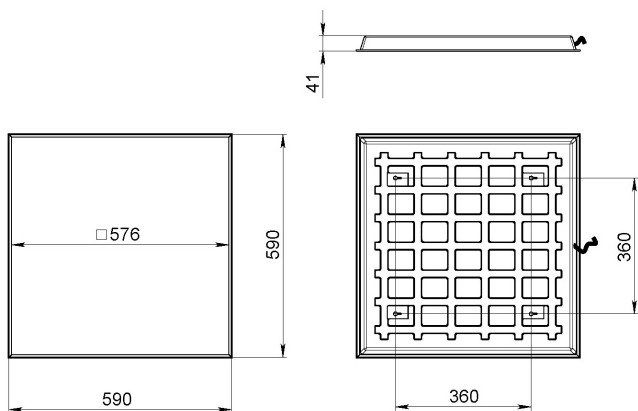
Рис.1 Габаритный чертёж.
