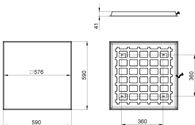
Рис.1 Габаритный чертеж.
