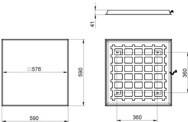
Рис.1 Габаритный чертеж.
