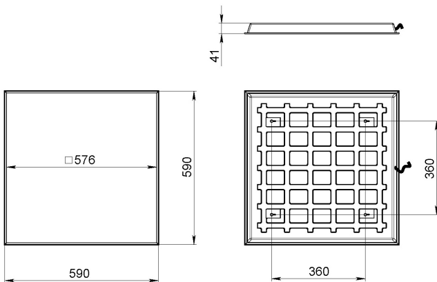
Рис.1 Габаритный чертёж.
