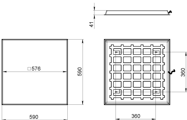
Рис.1 Габаритный чертёж.
