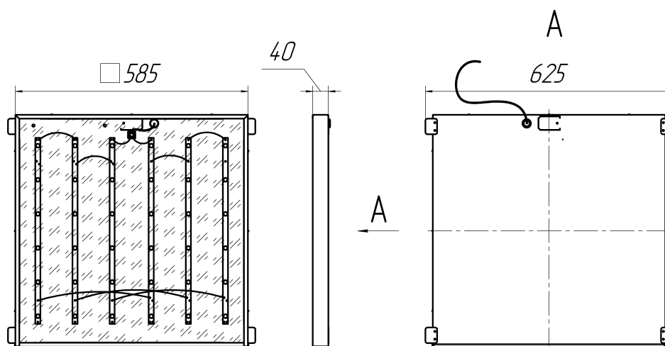
Рис.1 Габаритные размеры
