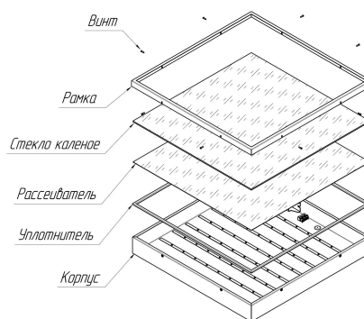
Рис. 2 Взрыв-схема..
