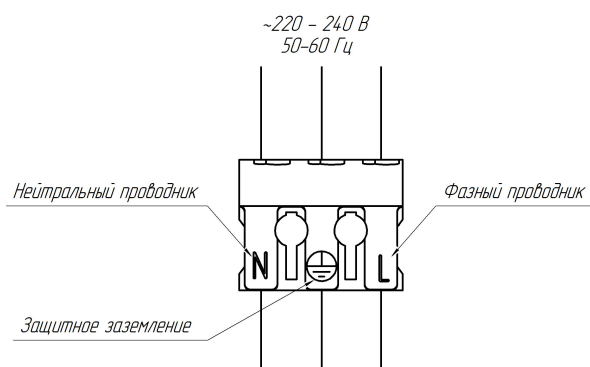
Рис. 3 Схема подключения.
