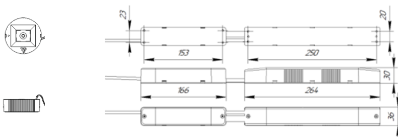
Рис. №3 Габаритный чертёж.
