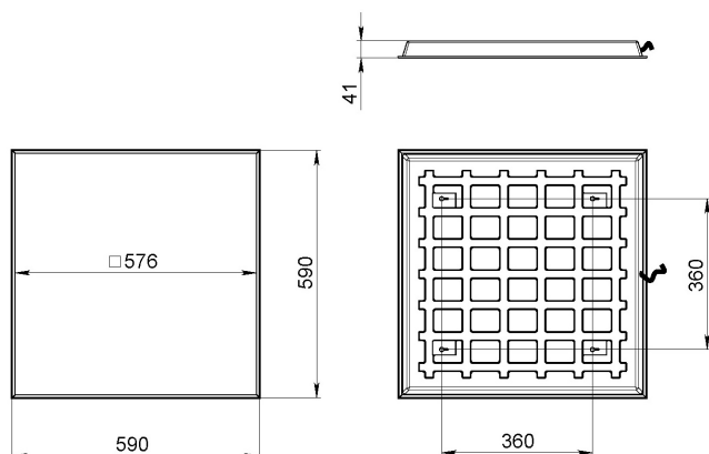
Рис.1 Габаритный чертеж.
