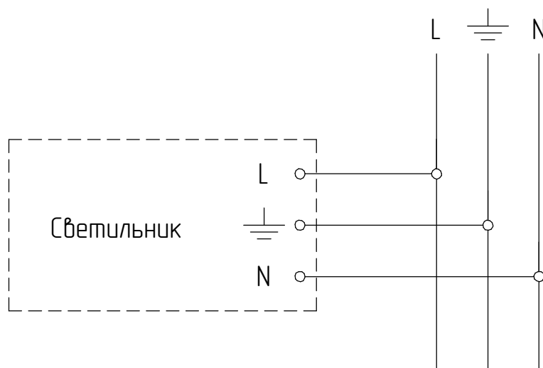
Рисунок 4 - Схема подключения светильника
