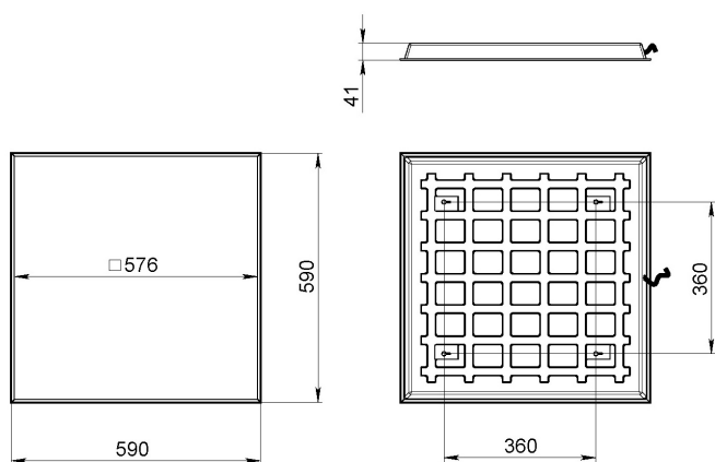
Рис.1 Габаритный чертеж.
