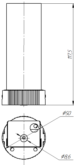
Рис. №2 Габаритный чертёж.
