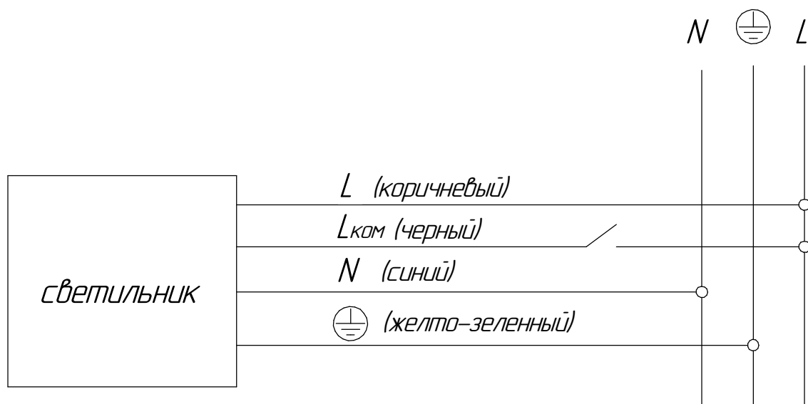
Рисунок 4 - Схема подключения светильника с БАП.
