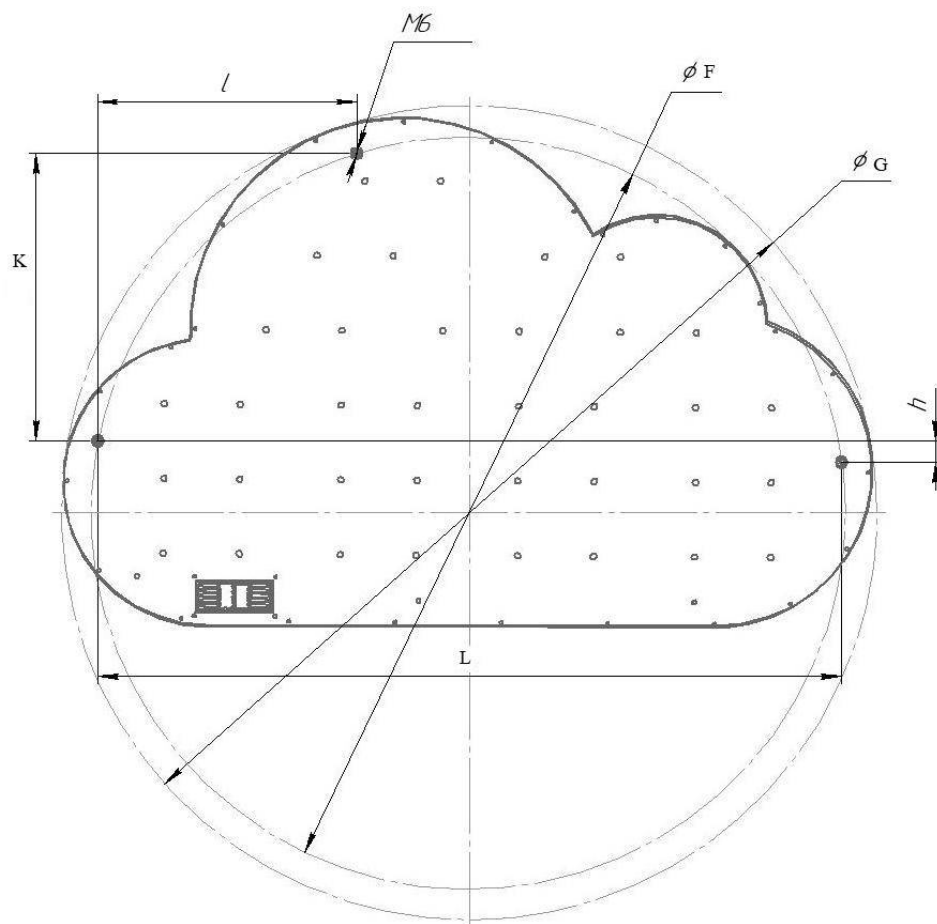
Рисунок 3 - Схема нанесения разметки для установки подвесов светильников
