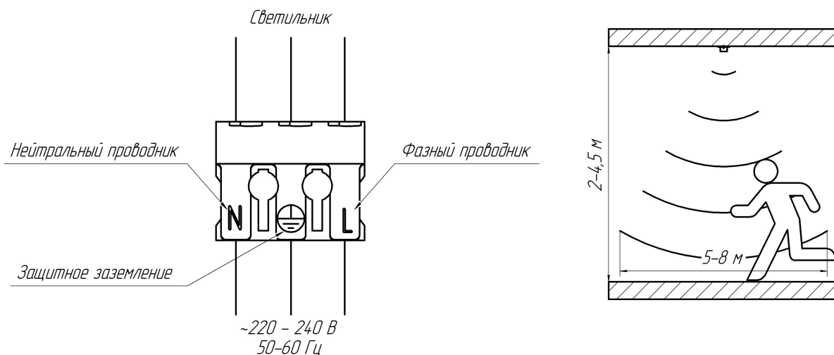
Рис. 2 Схема подключения.
