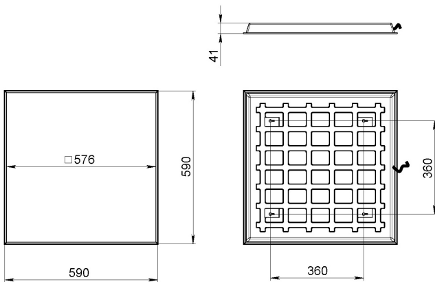
Рис.1 Габаритный чертёж.
