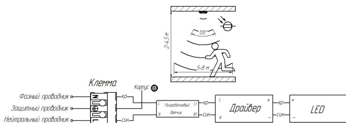
Рис.3 Принципиальная схема подключения с микроконтрольным датчиком.
