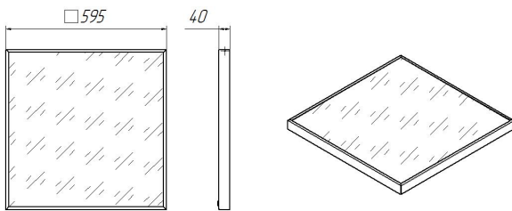
Рис.1 Габаритные размеры
