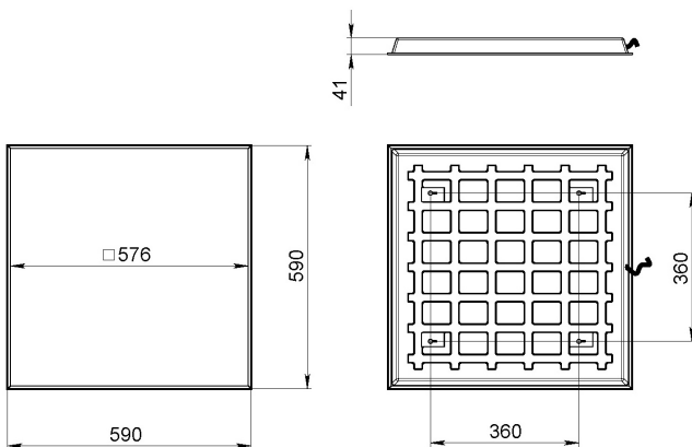
Рис.1 Габаритный чертеж.
