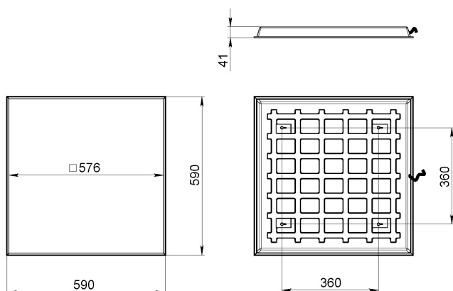
Рис.1 Габаритный чертеж.
