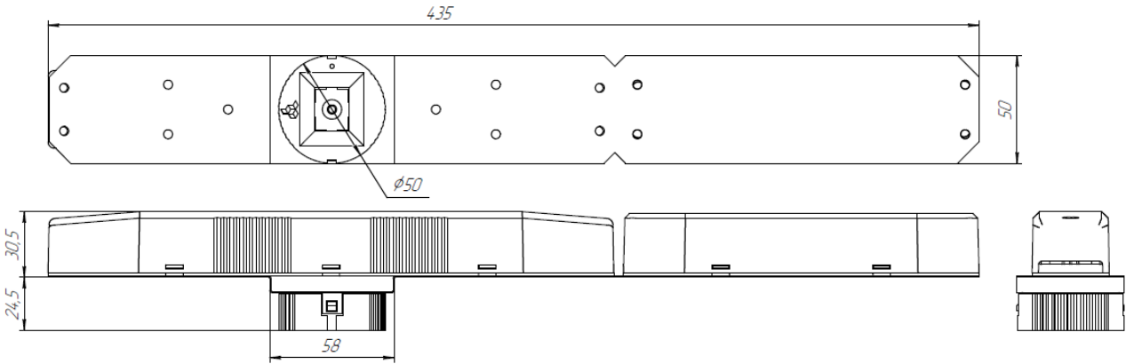
Рис. №2 Габаритный чертёж.
