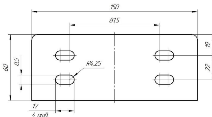
Рисунок 5 - Лира светильника (ДСП36-10, 35, 55 Вт).
