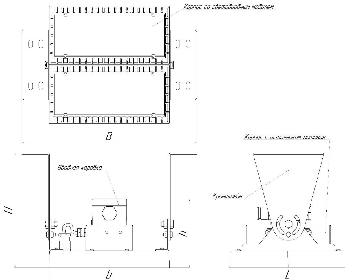
Рисунок 2 - Габаритные размеры светильника ДСП36-110, 160, 210, 270
