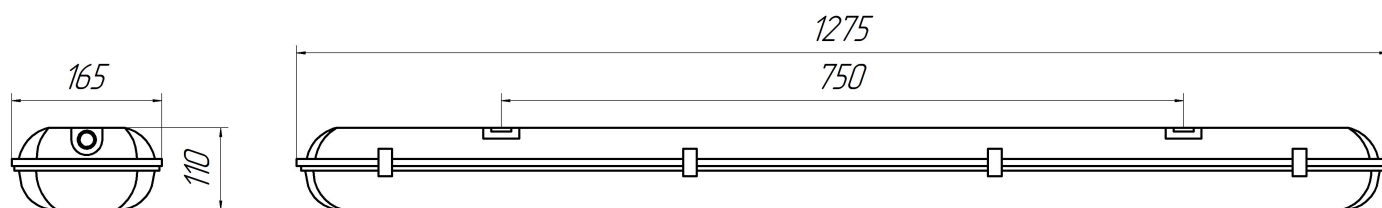
Рис. 1 Габаритный чертеж.
