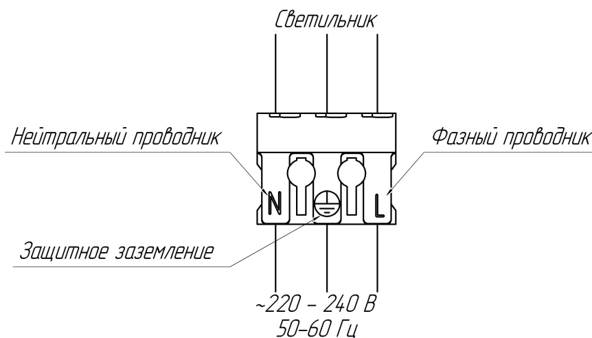
Рис. 2 Схема подключения.
