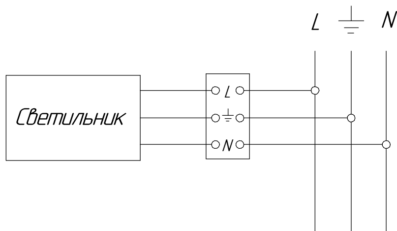
Рисунок 2.Схема подключения светильника к сети
