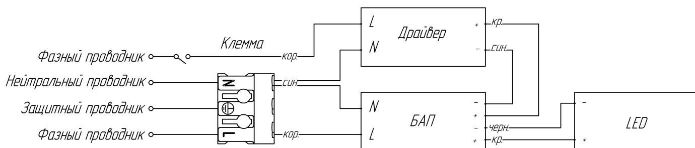
Рис. 2 Схема подключения.
