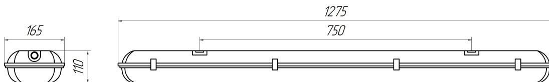
Рис. 1 Габаритный чертеж.
