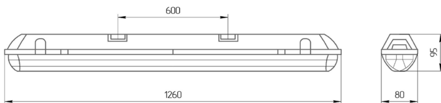
Рис. 1 Габаритный чертеж.
