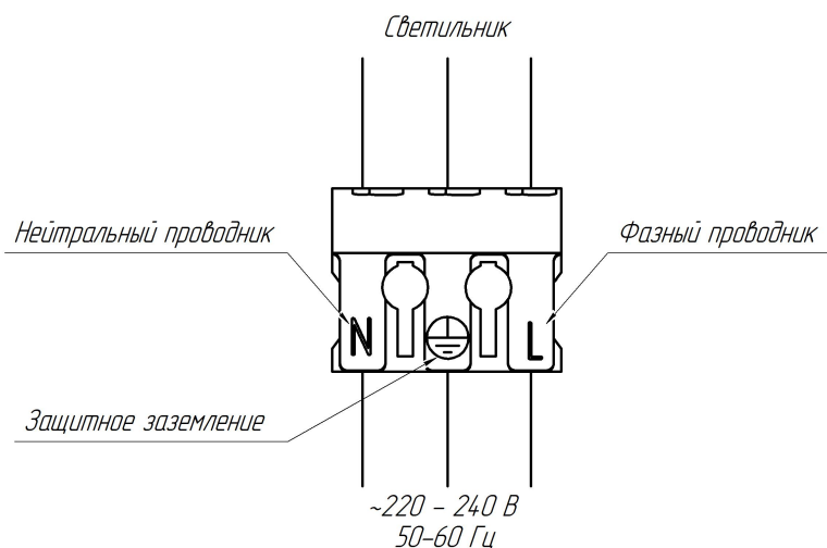
Рис. 2 Схема подключения.
