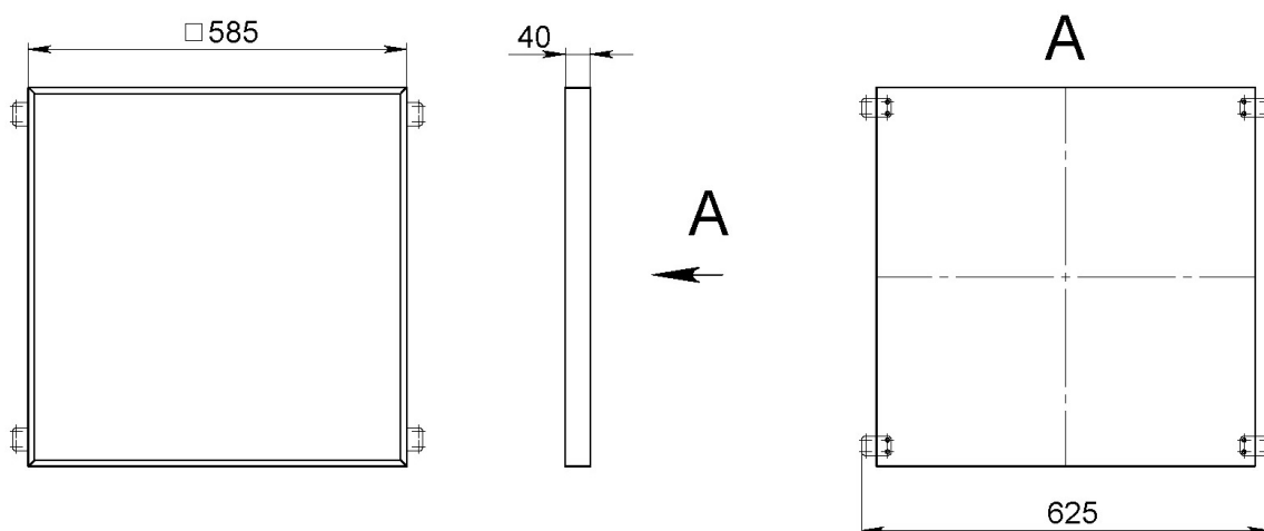
Рис.1 Габаритный чертеж.
