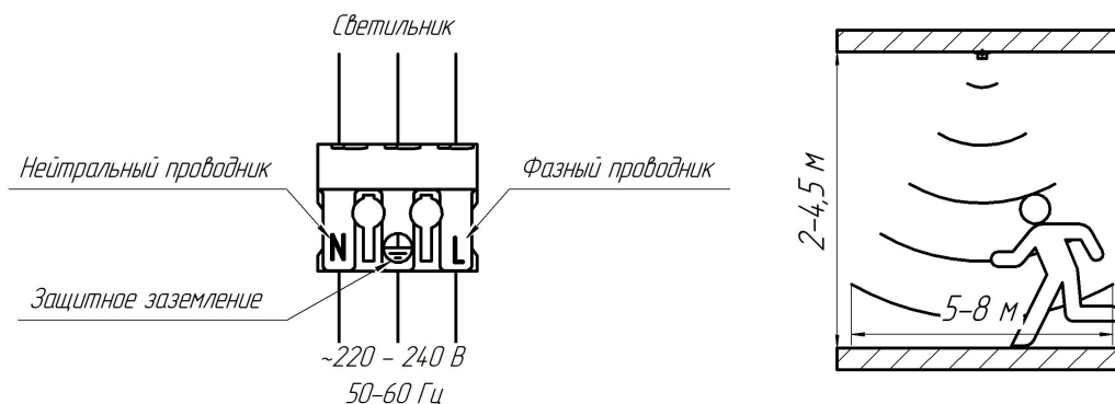
Рис. 2 Схема подключения.
