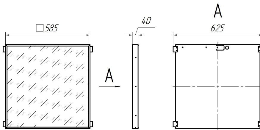
Рис. 1 Габаритный чертеж.
