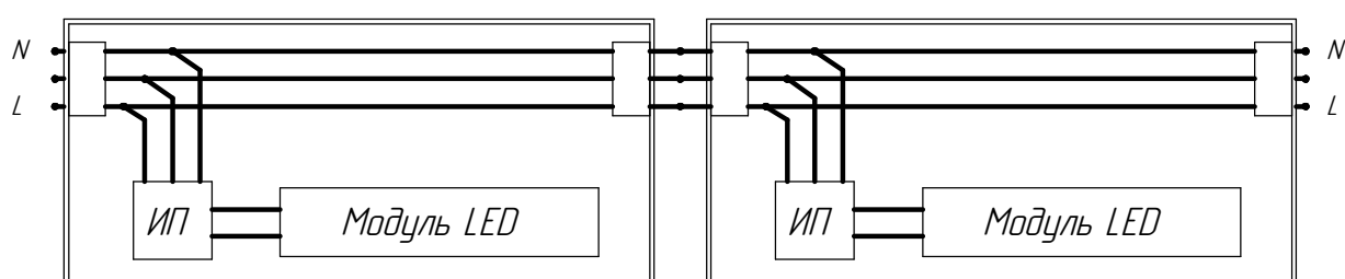
Рисунок 6 - Схема сквозной проводки
