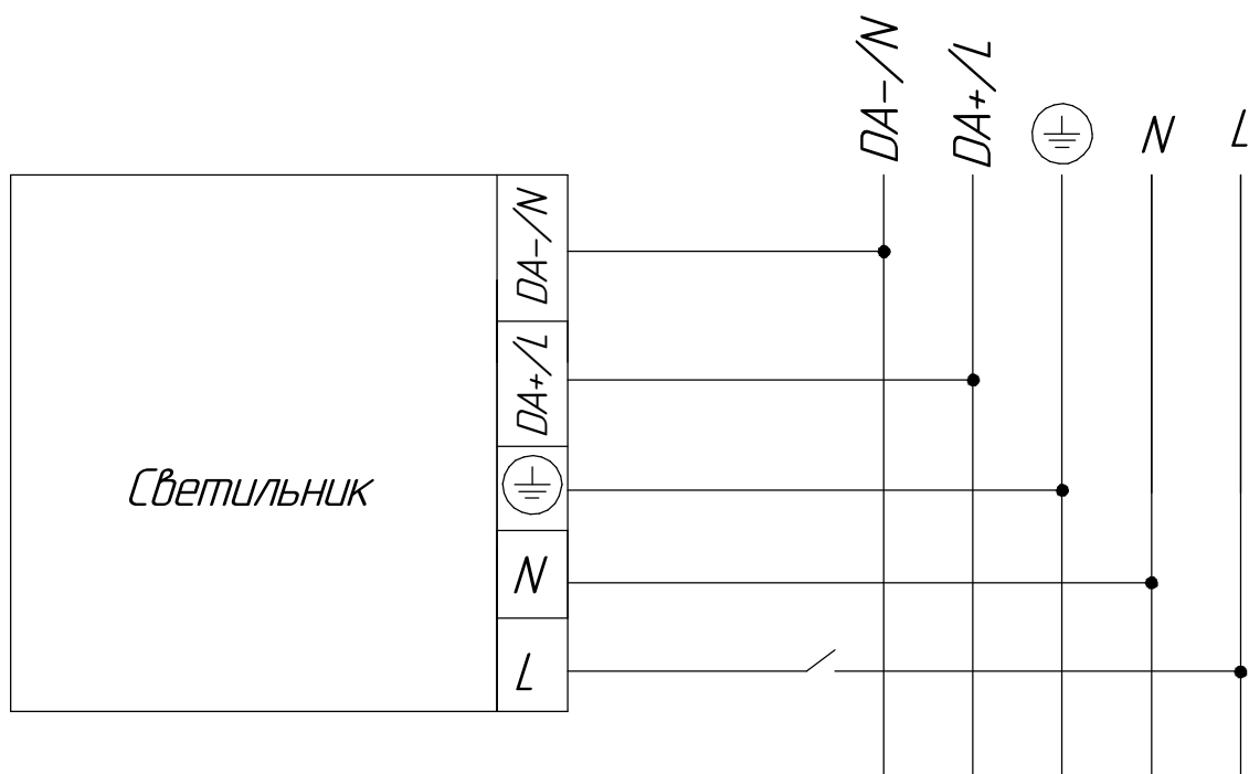
Рисунок 6 - Схема подключения светильника с управлением и с функцией Дежурный режим к электрической сети
