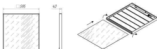
Рис.2 Габаритные размеры светильника с IP 20
