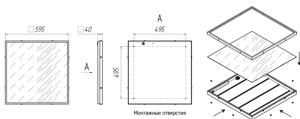
Рис.1 Габаритные размеры светильника с IP 54
