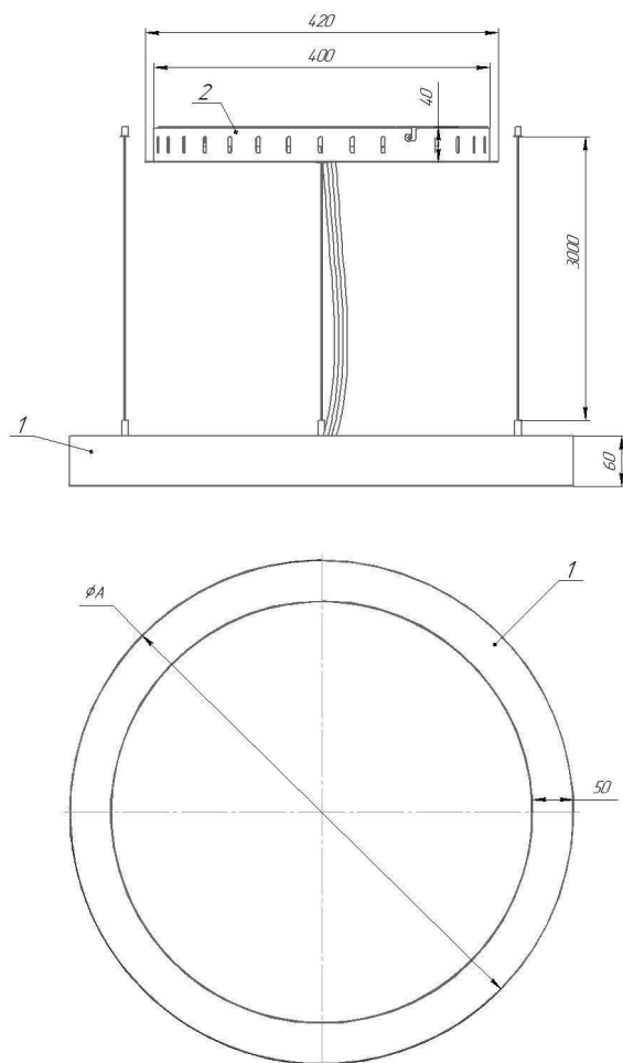
Рисунок 1 - Светильники серии ДСО33 Horizon Ring
