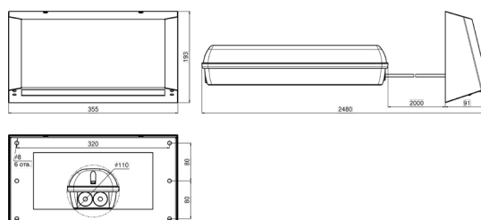
Рис. №2. Автономный аварийный светильник эвакуационного освещения с функцией TELECONTROL. Источник питания STABILAR
