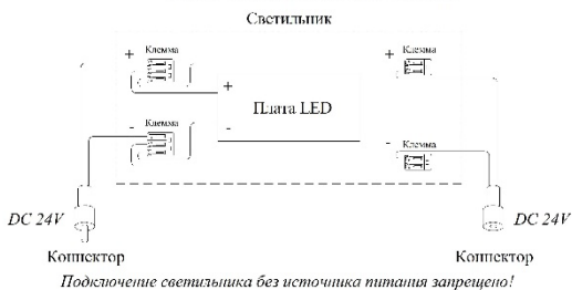
Рис.2 Монтажная схема
