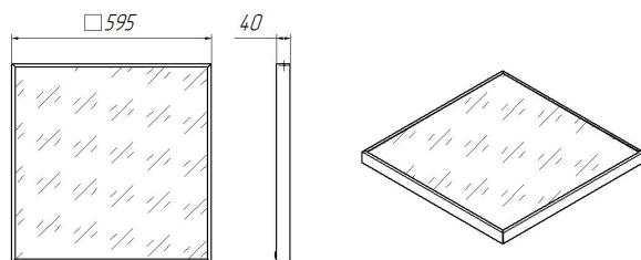
Рис.1 Габаритные размеры
