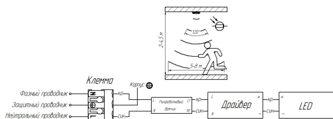
Рис.3 Принципиальная схема подключения с микроконтроллером датчиком.
