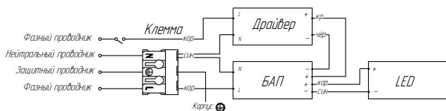
Рис.5 Принципиальная схема подключения с блоком аварийного питания.
